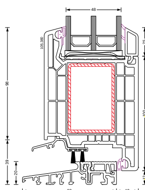
próg Alumaster Combi - 105.380
