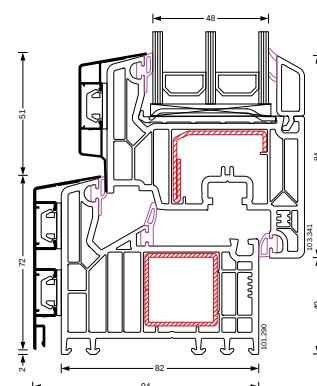
101.290 - 103.341 z nakładką ALU
